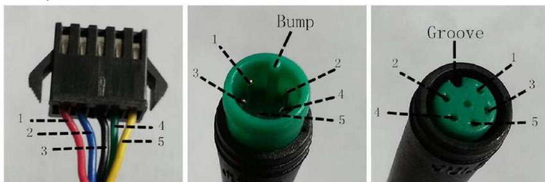
Connettore sul display
